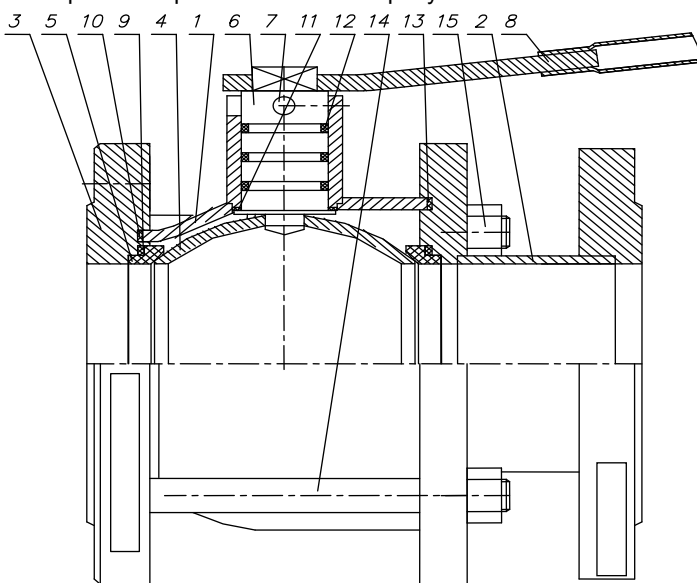
Рисунок 1. Общее устройство
